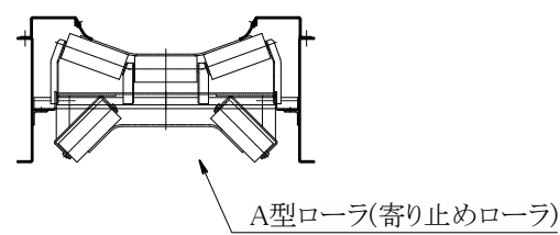
A-A断面 S=1/30
