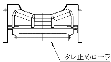
B-B断面 S=1/30
