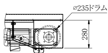
1.5kW中空軸ギヤモータ
