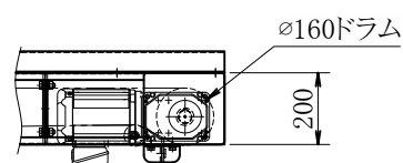
0.75kW中空軸ギヤモータ
